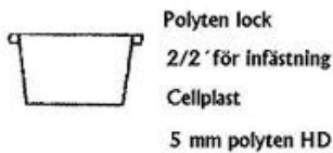
Rektangulär ponton
